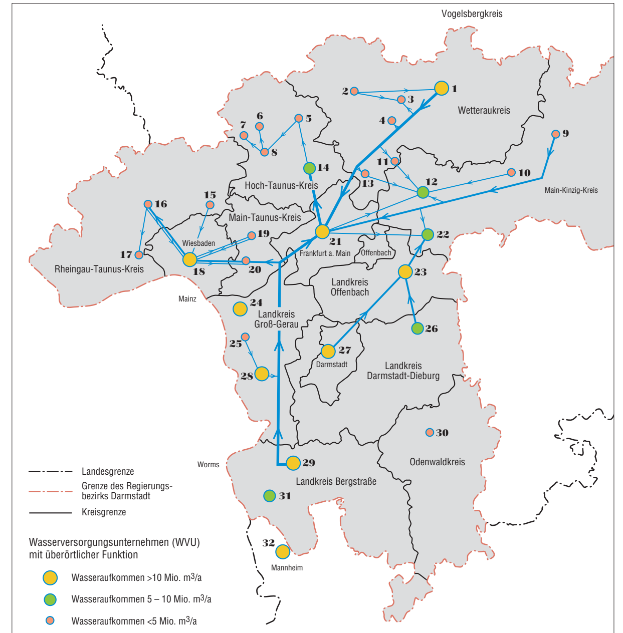
Abb. 17. Wasserverbund im Rhein-Main-Gebiet.
